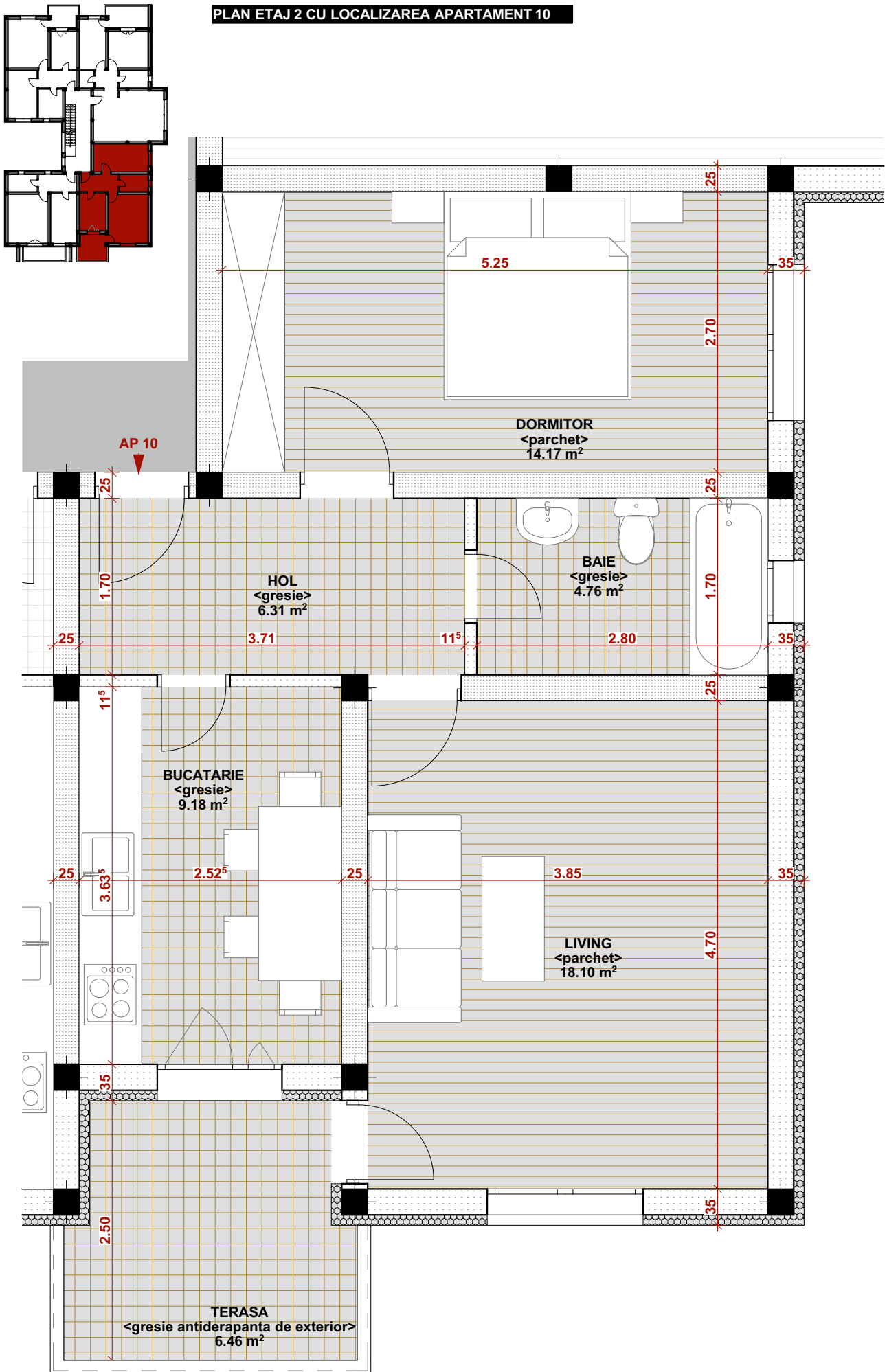
PLAN ETAJ 2. APARTAMENT 10 - Suprafata utila 52.52 mp, Suprafata terasa 6.46 mp
