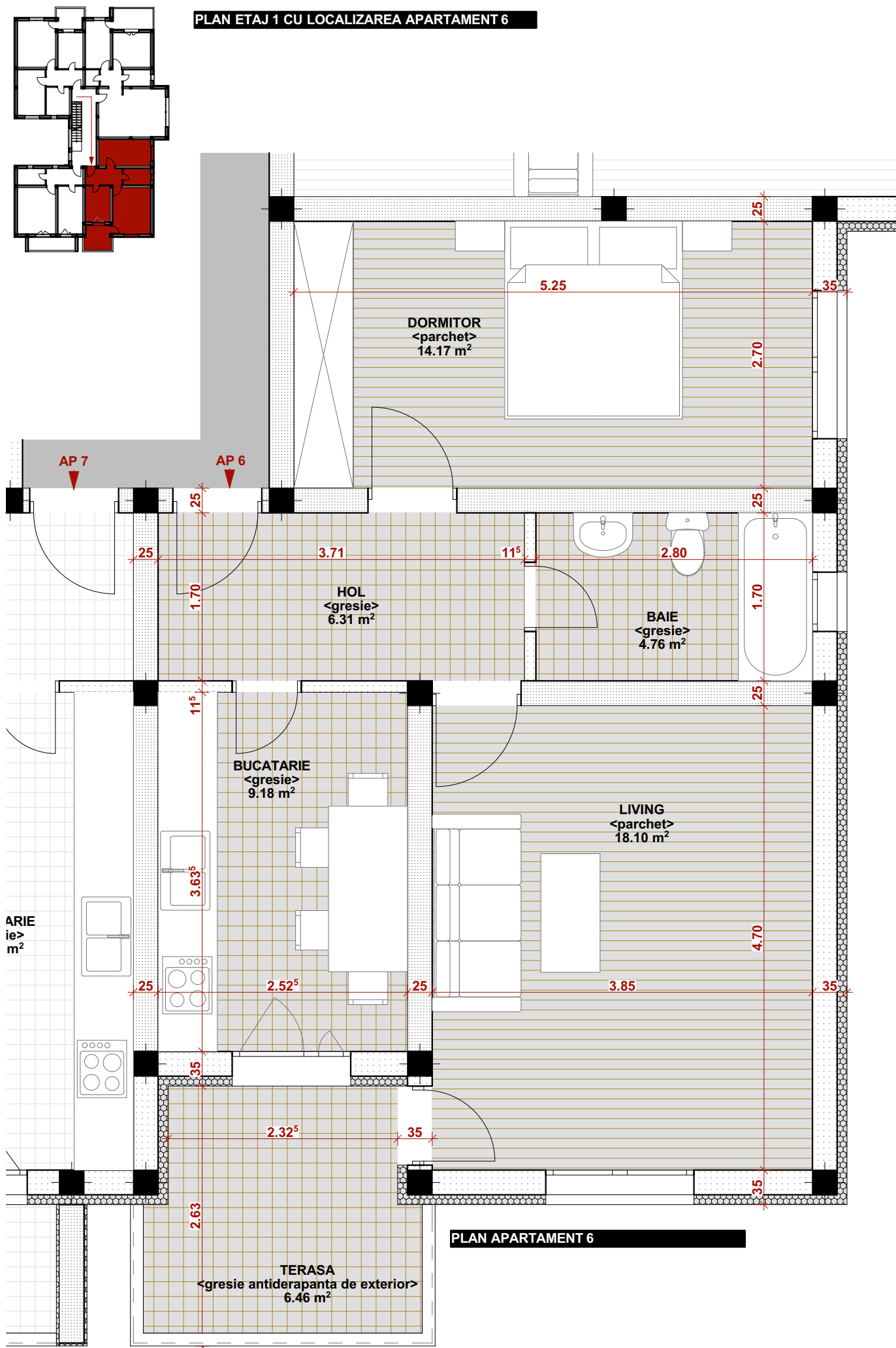
PLAN ETAJ 1. APARTAMENT 6 - Suprafata utila : 52.52 mp, Suprafata terasa 6.46 mp
