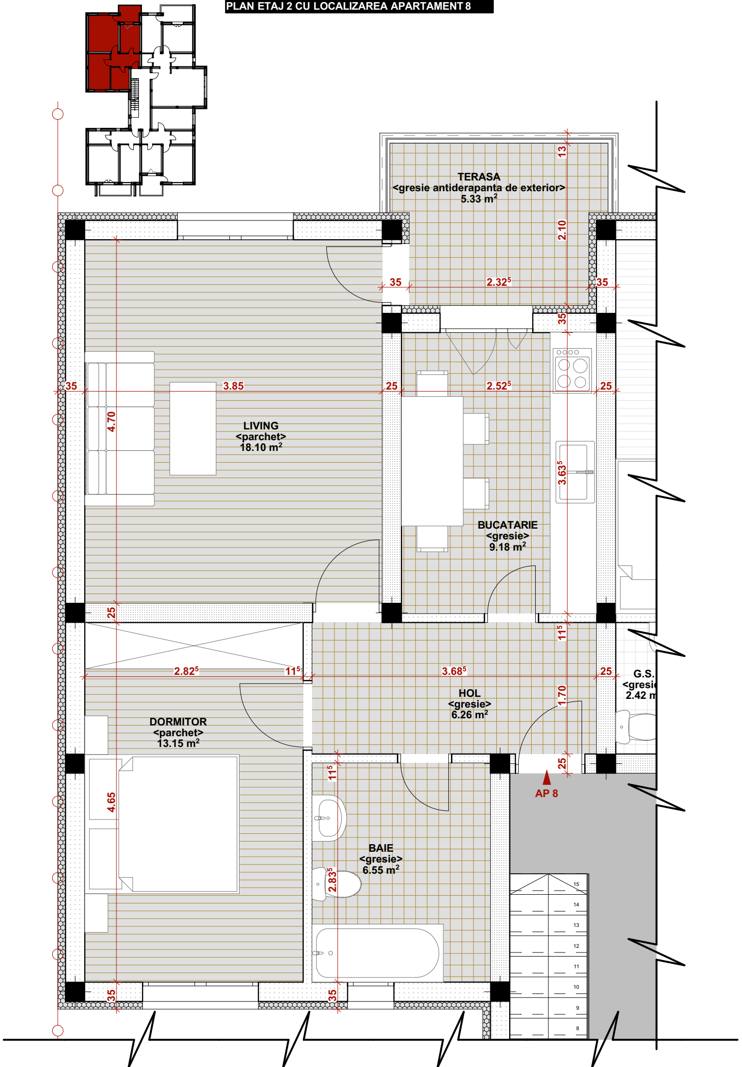
PLAN ETAJ 2. APARTAMENT 8 - Suprafata utila 53.24 mp, Suprafata terasa 5.33 mp
